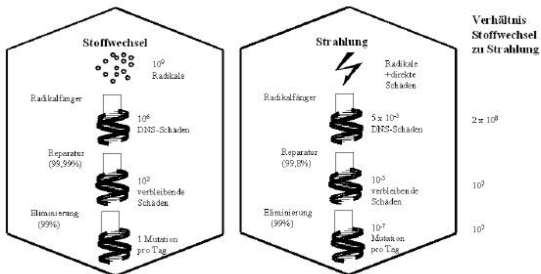
Abbildung: Vergleich von DNS-Schäden durch Stoffwechsel und durch Strahlung Angaben pro Zelle und Tag
